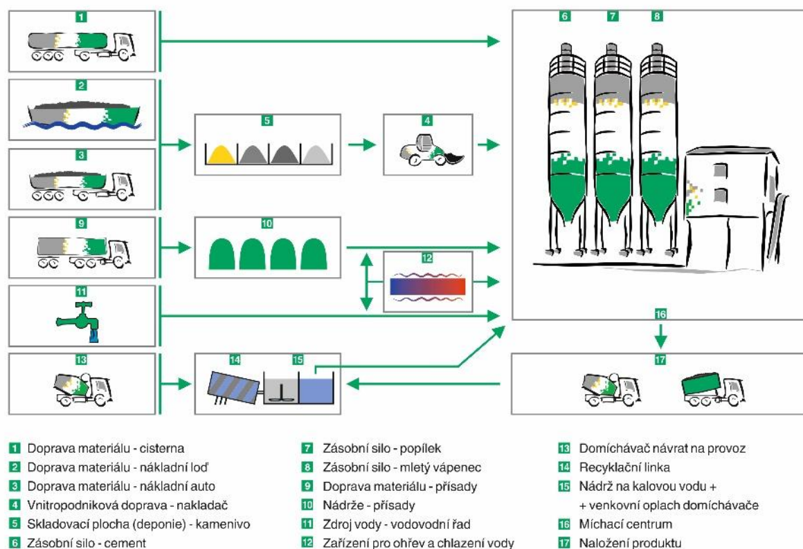
Obr.2: Schéma výrobního procesu
